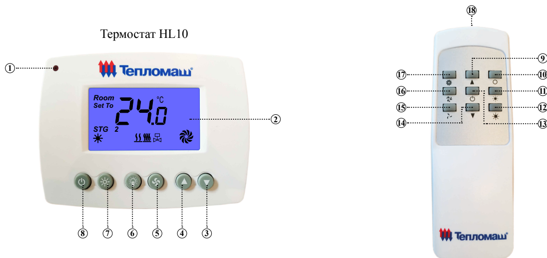
Дистанционный пульт управления HL
